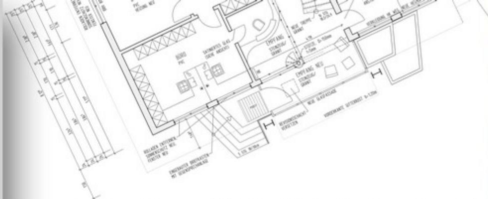
Um- und Aufbau Büro- und Sozialgebäude, Fa. Sinner, Kreuztal
