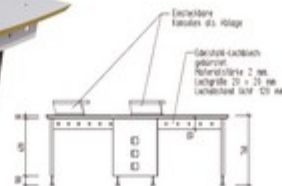
Schreibtisch Ansicht vorne M. 1:20
