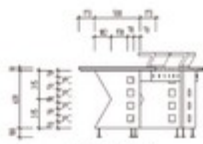
Schreibtisch Ansicht rechts M. 1:2
